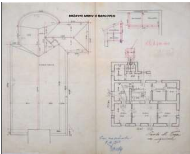
Slika 85. Tlocrt župne crkve, župnog stana i gospodarskih zgrada od 09.12.1913.
